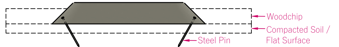
Elevation Scale 1:15
