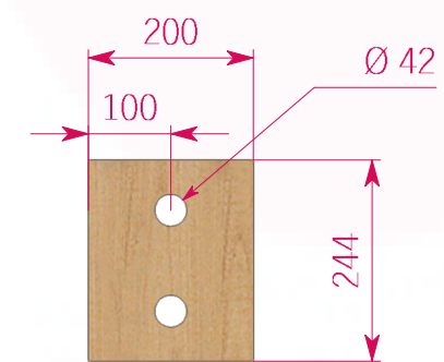
Template 17 Curve Seat Scale: 1:10
